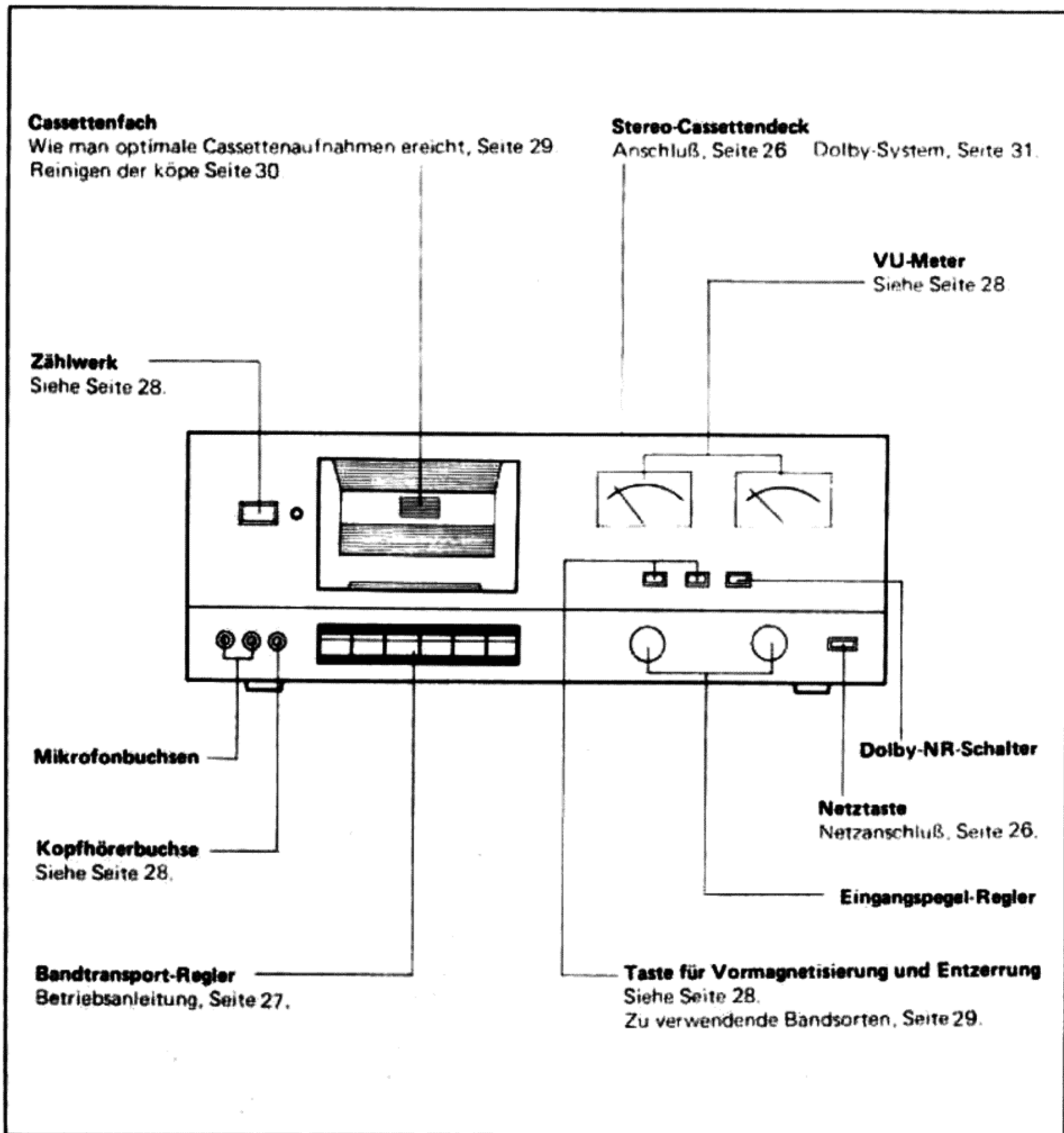
Abbildung 1. Hauptregler und Schalter
